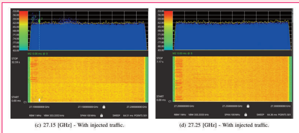
Figura 3: Spettri di segnale acquisiti in modalità Real Time nelle condizioni di rete scarica e di traffico forzato
