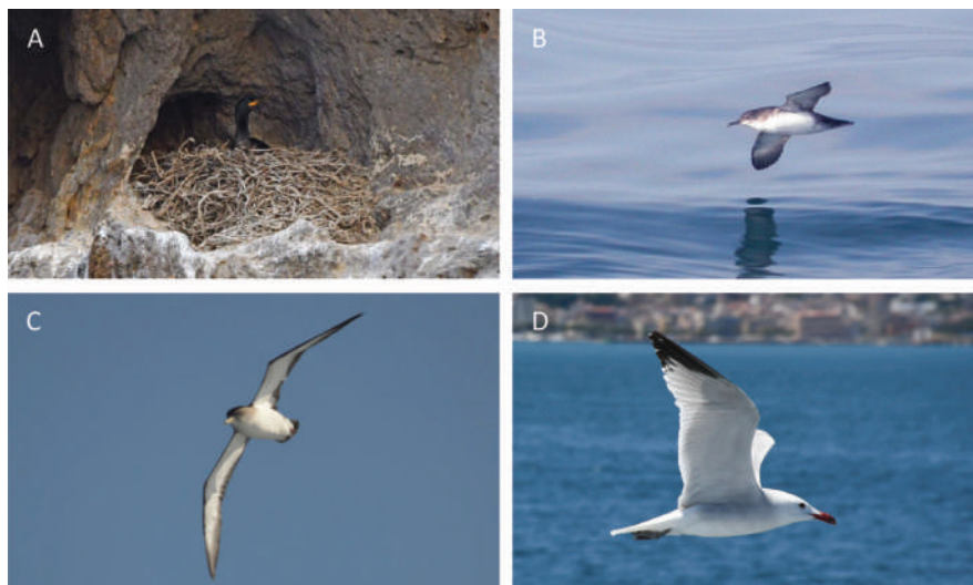
Figura 7. Immagini delle 4 specie di uccelli marini monitorati: A) Marangone dal ciuffo nel nido in cova; B) Berta minore in volo; C) Berta maggiore in volo; D) Gabbiano corso in volo
