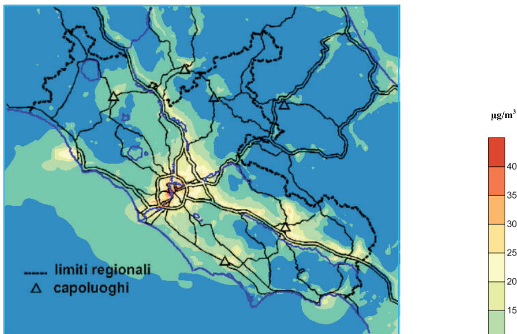
NO 2 MEDIA ANNUA 2023 Dominio del Lazio (1 km x 1 km)
