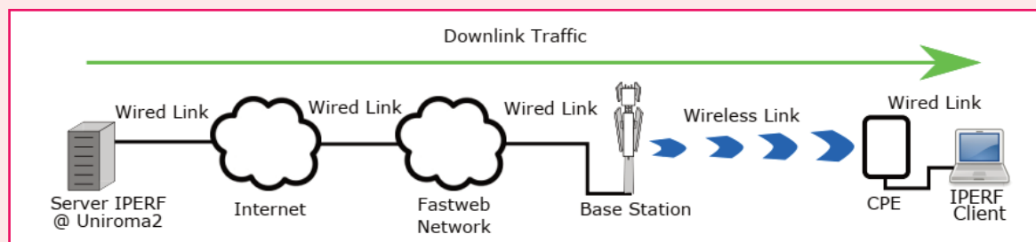
Figura 2: Schema a blocchi della configurazione client/server realizzata al fine di correlare le misure al traffico dati generato
