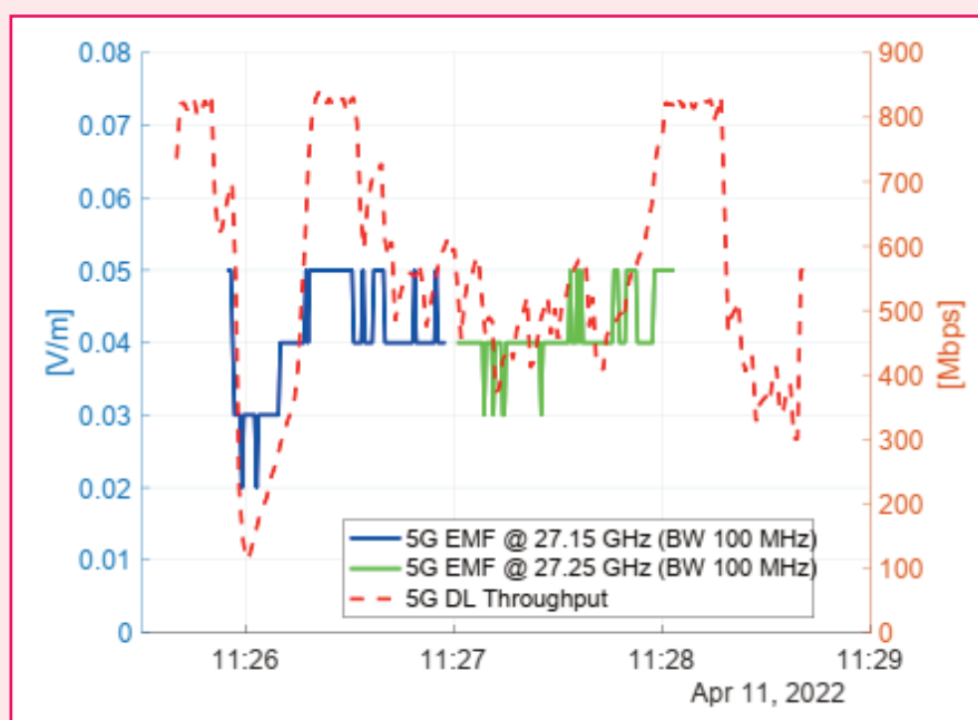
Figura 4: Livello di campo elettromagnetico misurato in funzione delle condizioni di traffico dati
