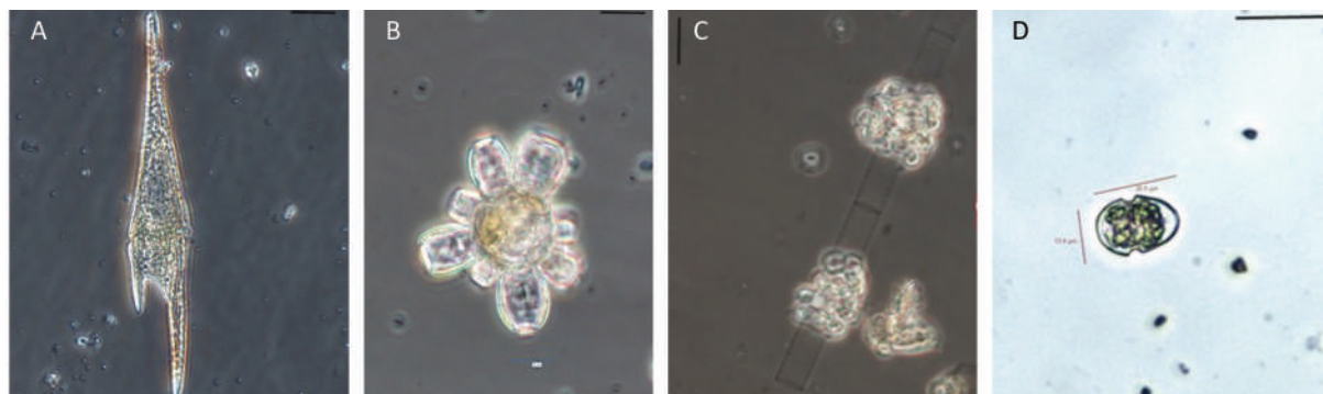
Figura 2. Immagini acquisite al microscopio ottico invertito di alcune specie di fitoplancton rinvenute nel 2023. A) Tripos furca (gruppo Dinoflagellati); B) Scyphosphaera apsteinii (gruppo Altro fitoplancton); C) Leptocylindrus mediterraneus (gruppo Diatomee); D) Heterocapsa niei (gruppo Dinoflagellati). Barra micrometrica = 20 \mu\text{m}
