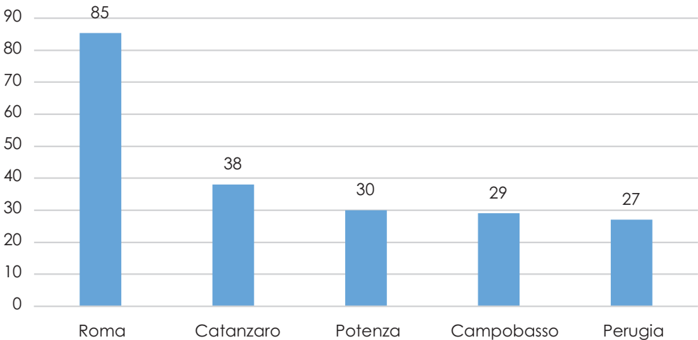
Indice di durata dei periodi di caldo WSDI anno 2021 CLINO 1971-2000
